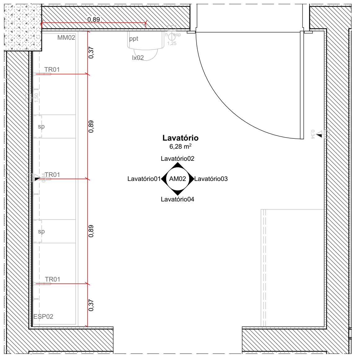
Pavimento Térreo 1:20
