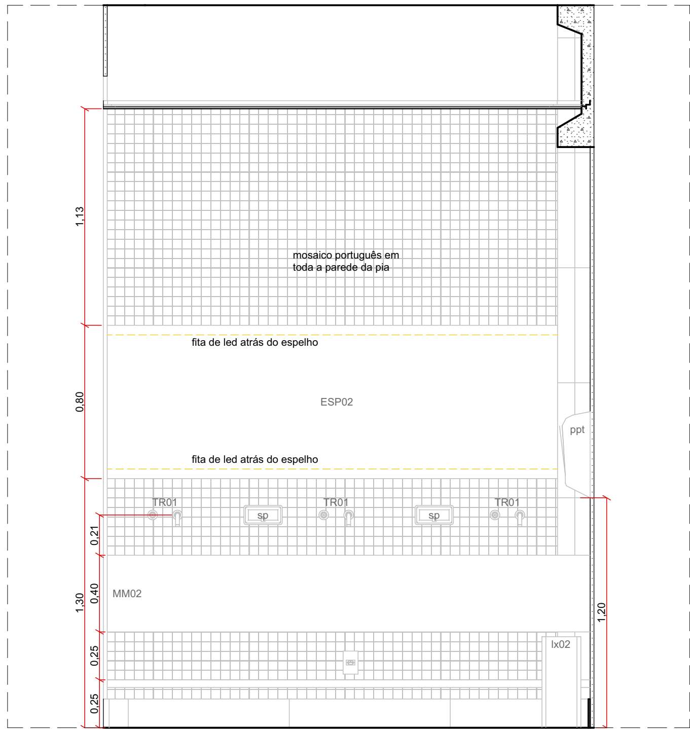
Lavatório01 1:20
