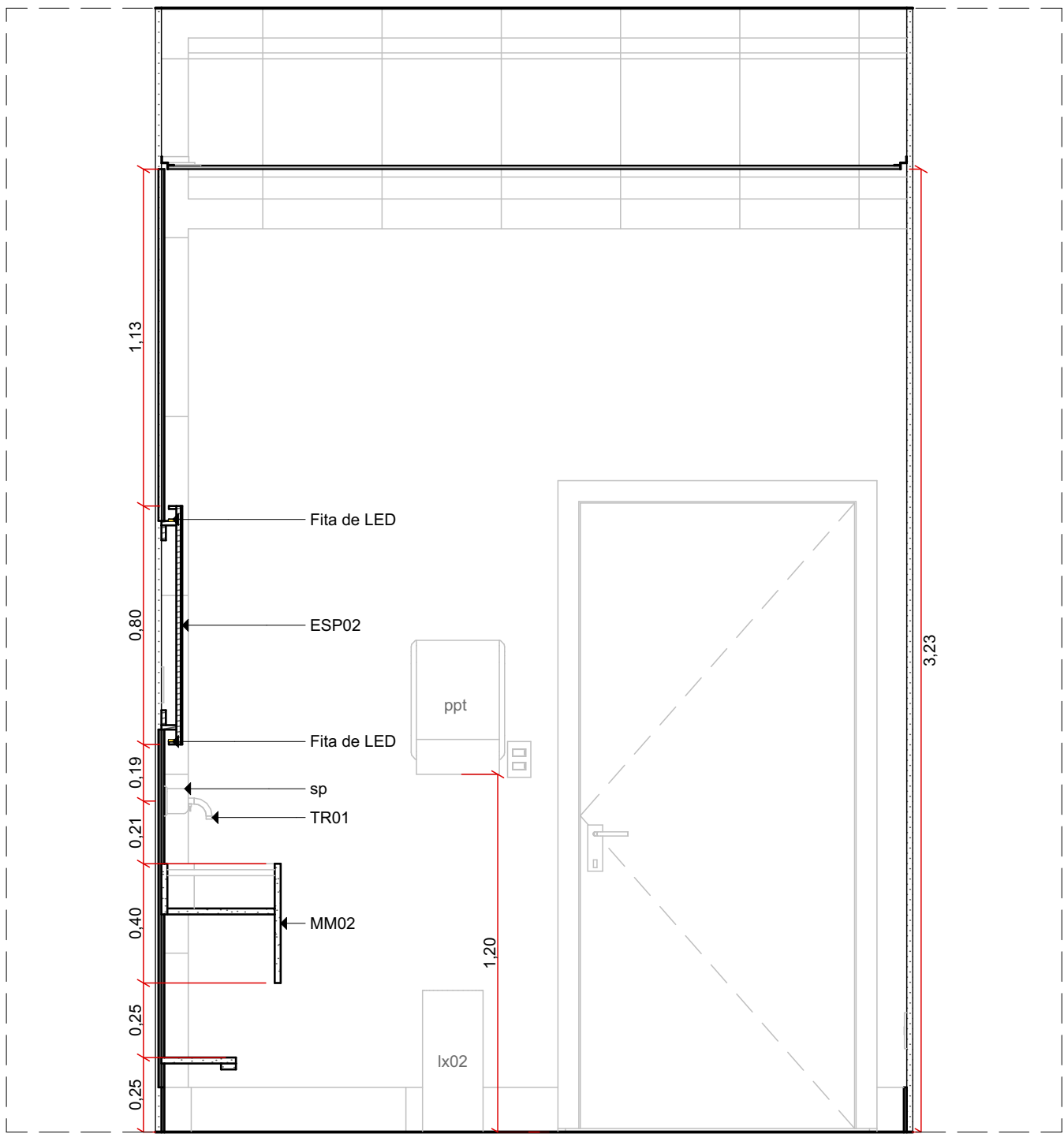
Lavatório02 1:20
